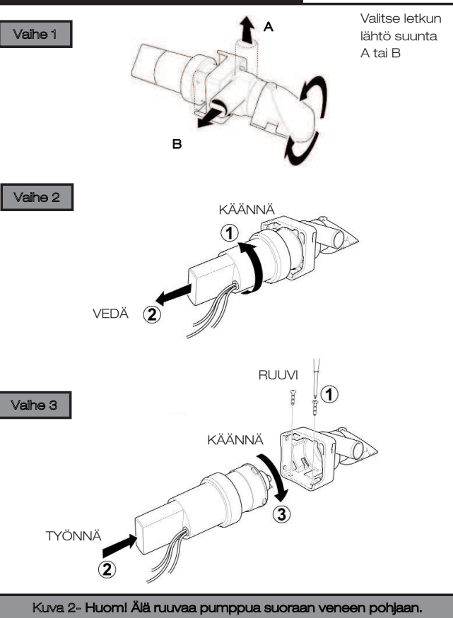
Kuva 2- Huom! Älä ruuvaa pumppua suoraan veneen pohjaan.
