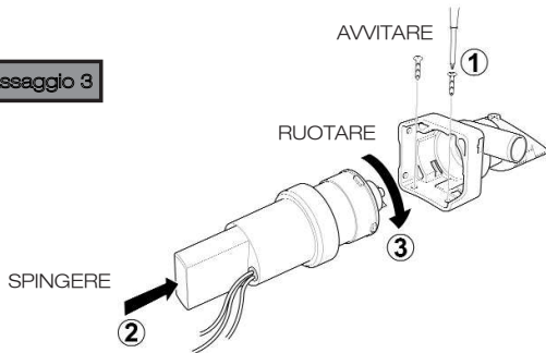
Figura 3 NON avvitare direttamente allo scafo
