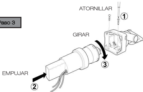
dibujo 3- No atornille la bomba directamente al casco
