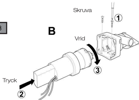
Bild 2- Pumpen skall inte skruvas direkt på skrovet
